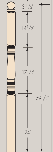
FH4506
