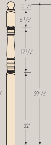
FH4501
