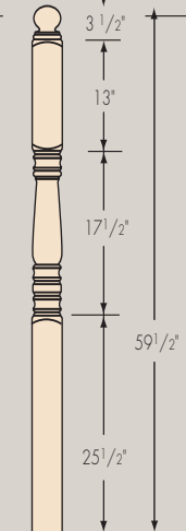
FH4505
